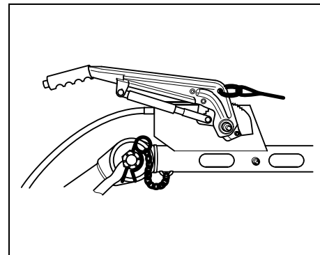
Рычаг ручного тормоза в нижнем положении – тормоз не работает
