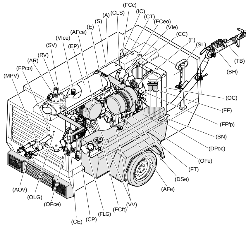
XAVS 166 Dd и XAHS 186 Dd с некоторыми опциями
